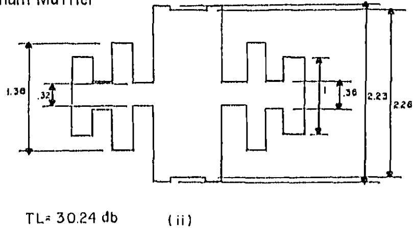
Optimum Muffler
