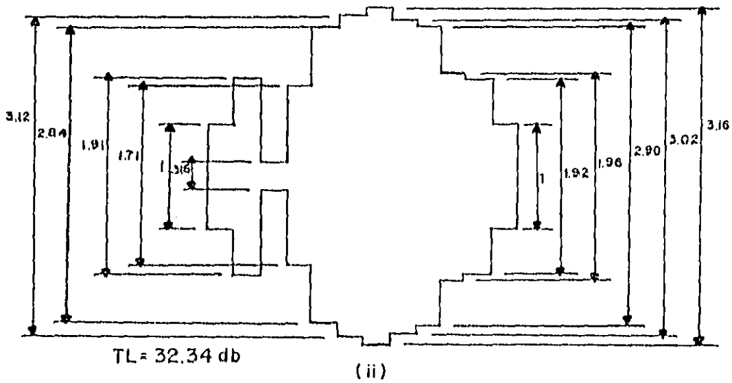
Optimum Muffler
