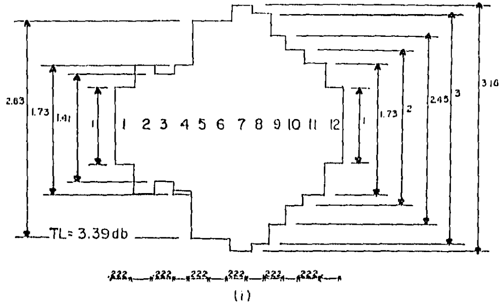
Optimum Muffler
